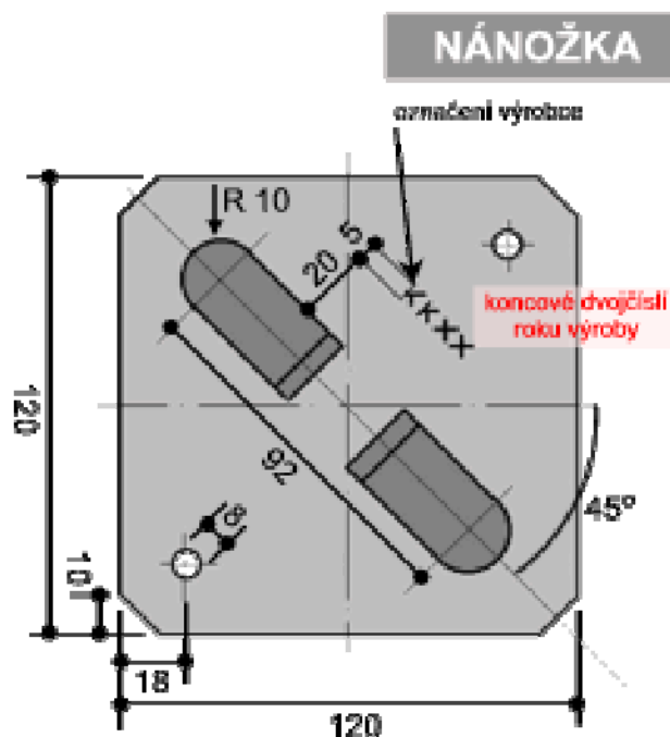
Obr.3 – Nánožka
