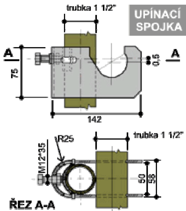
Obr.1 - Upínací spojka 40
