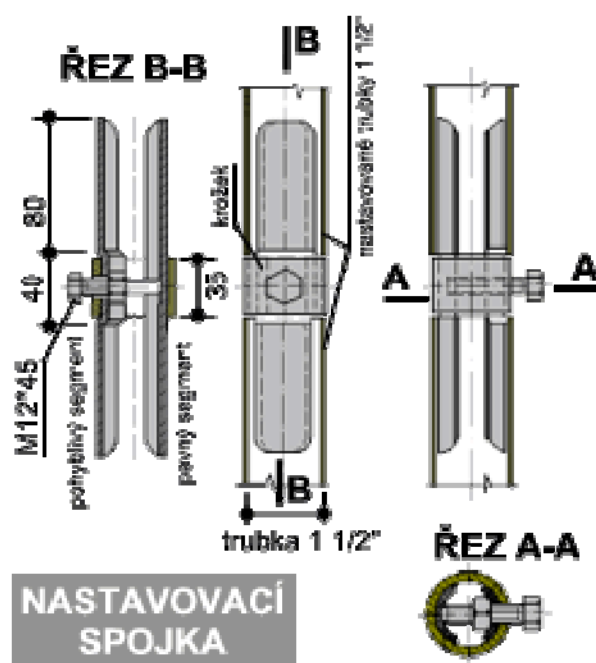
Obr.2 - Nastavovací spojka 40
